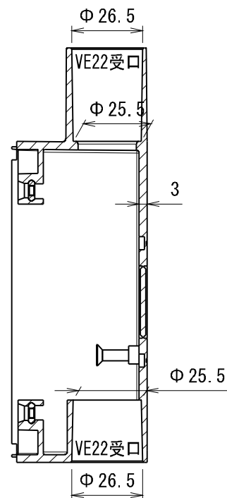
断面 A-A
